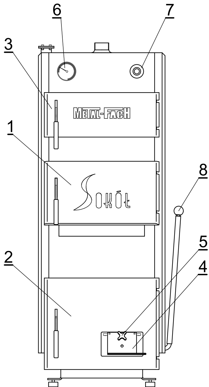
Рисунок 7.1 Основные элементы конструкции котла SE MAX
