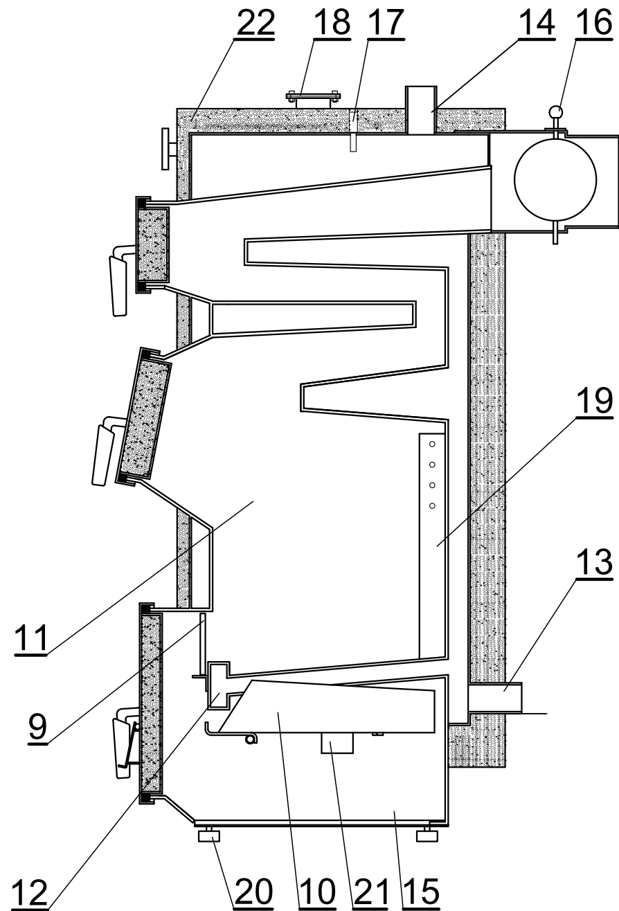
Рисунок 7.1 Основные элементы конструкции котла SE MAX
