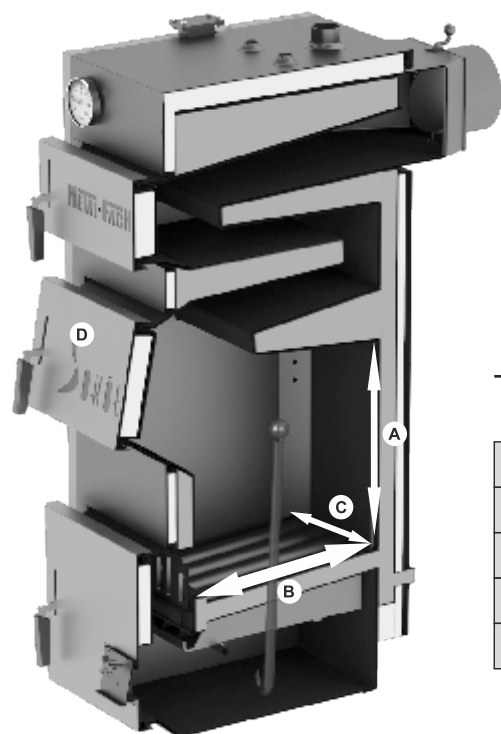
Рисунок 7.2.2 Размеры запасной топочной камеры и загрузочного отверстия SE MAX
