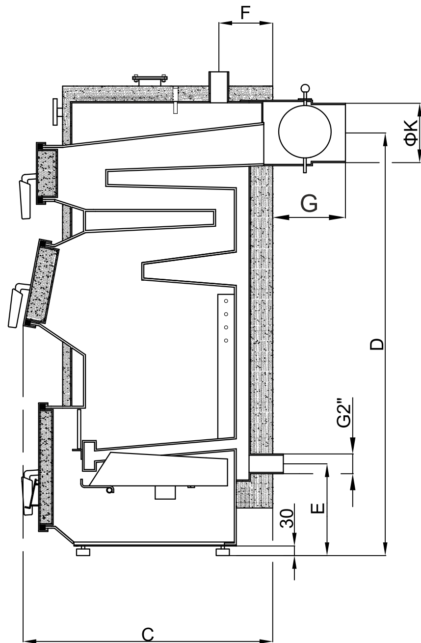
Рисунок 7.2.1 Размеры котла SE MAX
