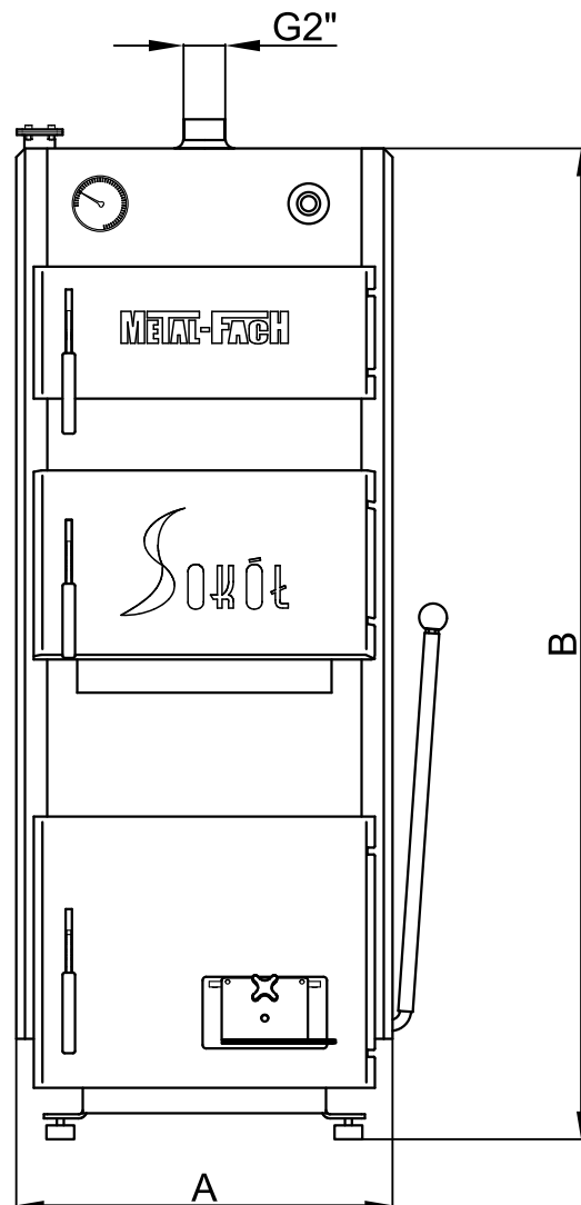
Рисунок 7.2.1 Размеры котла SE MAX
